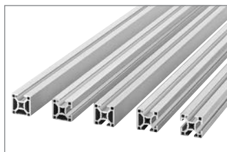
Profilati scanalatura 8 mm, modulo 30 mm (pag. 2-15)
